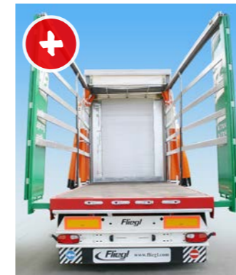
Maximaler Zugriff auf die Ladefläche: Mit Heckrungenverbreiterung und Schiebeverdeck werden auch sperrige Güter unkompliziert be- und entladen.
